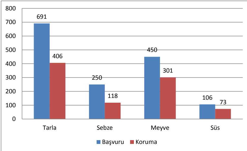
Grafik 6: Bitki gruplarına göre başvuru ve korunan çeşit sayıları. 31.12.2016
